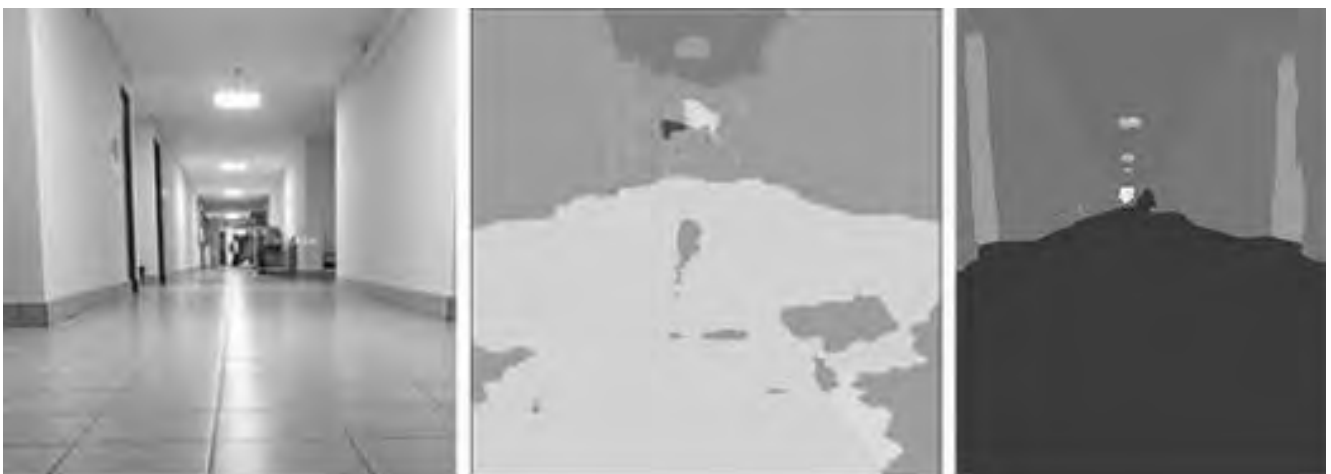
Fig. 5. Recognizing obstacles in the corridor of ACS department using: a – SSD classifier; b – UNET segmentation; c – Deeplab segmentation / Розпізнавання перешкоди в коридорі кафедри АСУ за допомогою: а – класифікатора SSD; б – сегментації UNET; в – сегментації Deeplab
