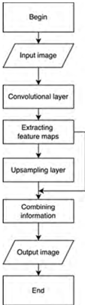
Fig. 1. Block diagram of the UNet model operation algorithm / Блок-схема алгоритму роботи моделі Unet
