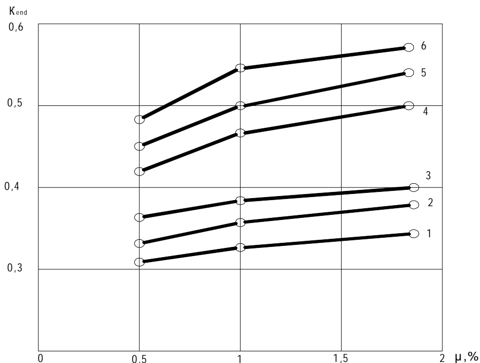
Рис. 2. Залежність коефіцієнта витривалості сірчаного склофіробетону від довжини фібри і процента армування: 1–3 – немодифікована сірка, довжина фібр відповідно 10; 30 і 50 мм; 4–6 – модифікована 5 % дциклопентадієну
