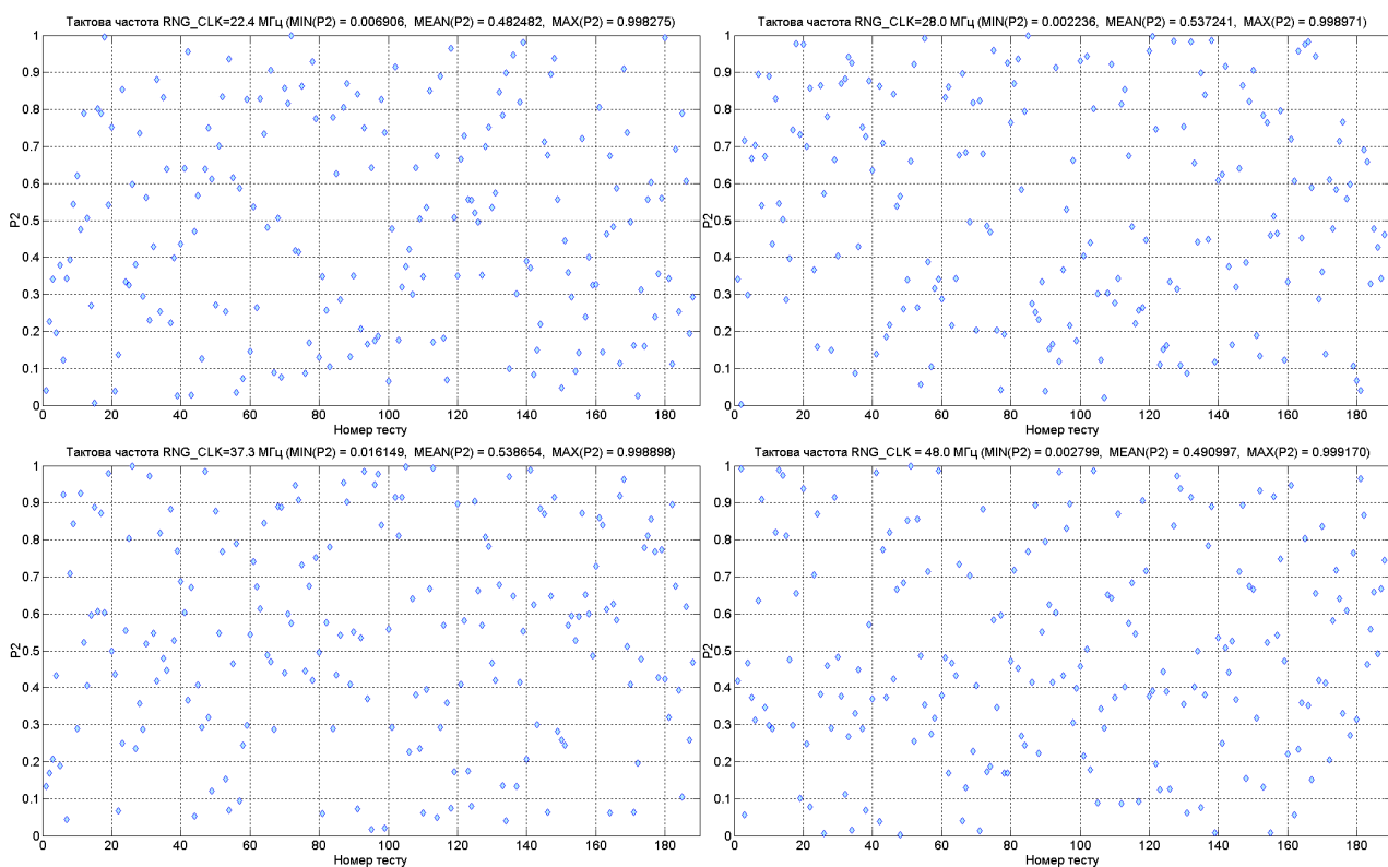
Рис. 5. Результати проходження тестів NIST STS згідно зі стратегією 2
