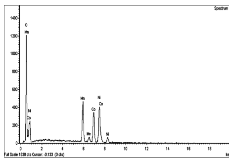
Fig. 2. EDAX spectrum of Li[Ni 0.5 Co 0.25 Mn 0.25 ]O 2 powder
