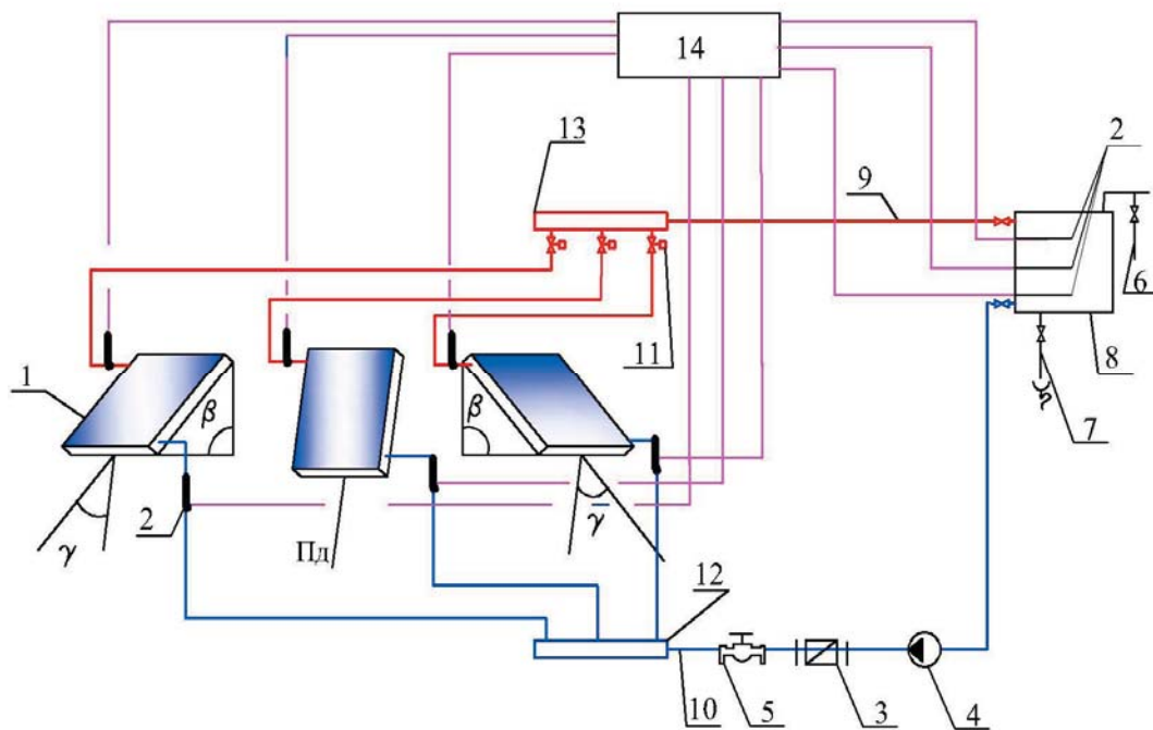
Рис. 1. Схема експериментальної установки: 1 – сонячний колектор; 2 – місце встановлення термометра; 3 – витратомір; 4 – насос; 5 – балансовий вентиль; 6 – патрубок відбору теплоносія; 7 – патрубок подачі холодного теплоносія або його зливу; 8 – бак-акумулятор; 9 – трубопровід подачі нагрітого теплоносія; 10 – трубопровід охолодженого теплоносія; 11 – вентиль; 12, 13 – гребінка; 14 – регулятор-вимірювач
