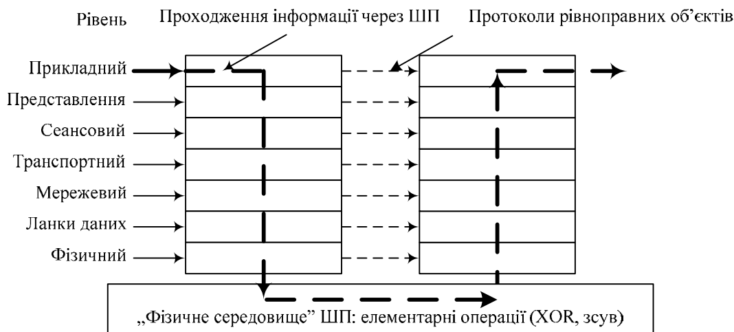
Рис. 3. Структура шифропроцесора
