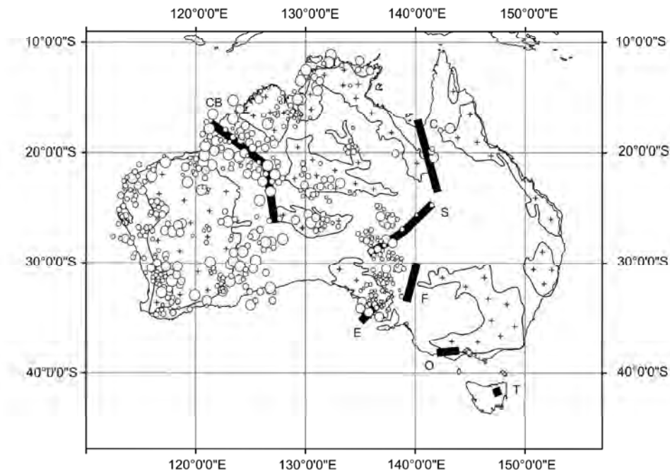
Рис.1. Карта Австралии [Национальная...2005], эпицентров землетрясений [Борисенко, Сафронов, 1993] и региональных аномалий электропроводности [Woods, Lilley, 1979; Kulik, 2004]. Названия аномалий электропроводности: С, Carpentaria; СВ, Canning Basin; Е, Eyte; F, Flinders; О, Otway; Т, Tarnar; S, south-west Queensland
